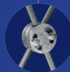
Kreuzklemme Knotenpunktverbindung zur Stabilisierung der Seile
